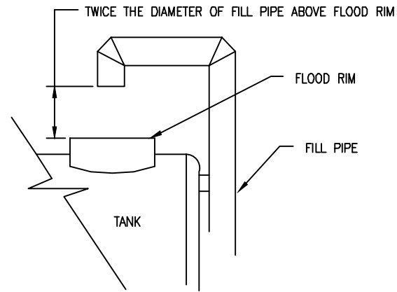
FILL PIPE DETAIL
